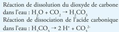
Doc. 3 Réaction de dissolution du dioxyde de carbone dans l'eau.
